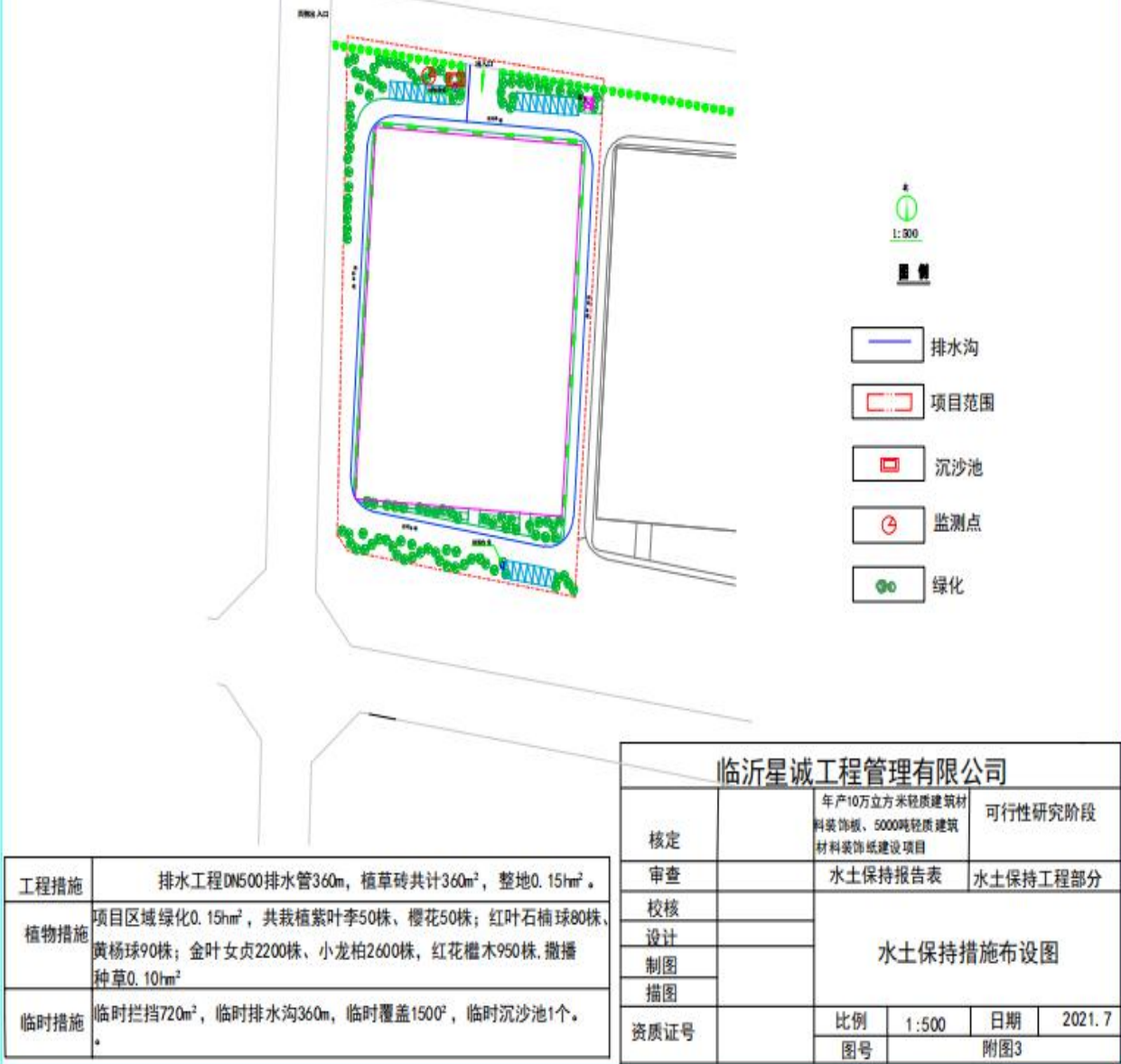
附图 3 项目分区措施总体布置图
